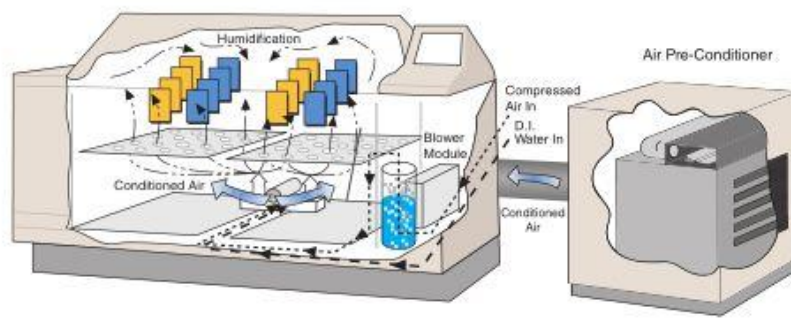
Q-FOG® CRH循环腐蚀盐雾箱可进行相对湿度控制。 中国腐蚀与防护网
